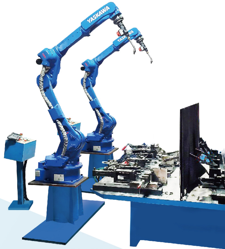
轉盤迴轉定位台 Rotational Positioning Table
