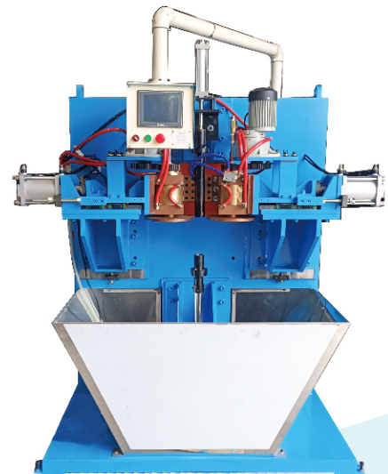
自動雙輪銲機 Automatic Twin-Wheel Welding Machine
