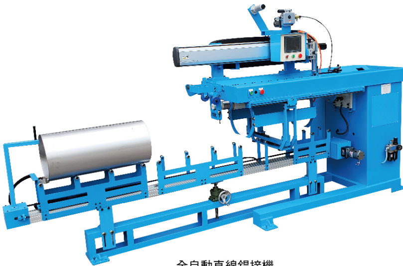
全自動直線銲接機 Automatic Seam Welder
