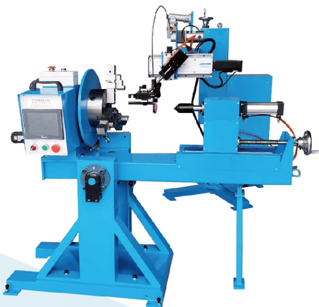
立/臥式二用銲接機 Vertical / Horizontal Positioner
