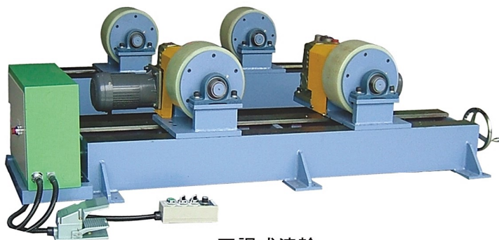
可調式滾輪 Adjusting Roller
